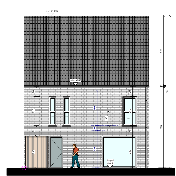
Voorgevel LOT 78
