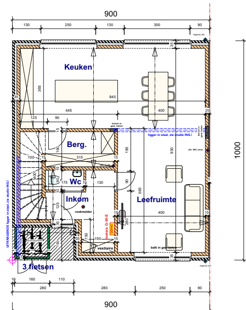
Gelijkvloers LOT 78
