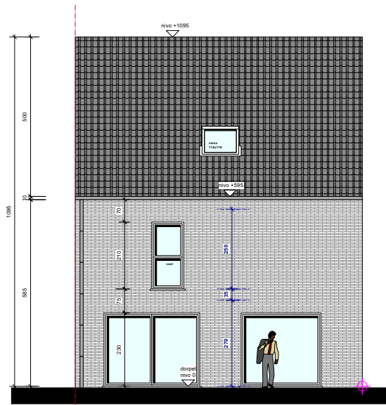
Achtergevel LOT 78
