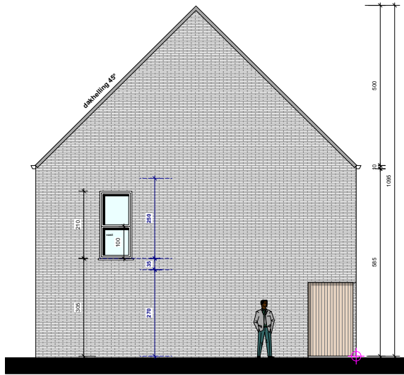
Zijgevel links
